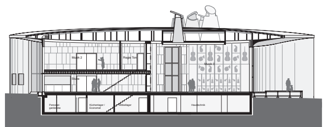
Schnittzeichnung Klanghaus (Meili & Peter Architekten AG)
